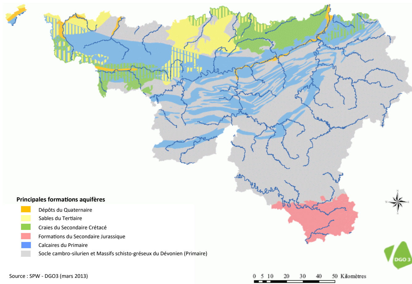
Principales formations aquifères de Wallonie
